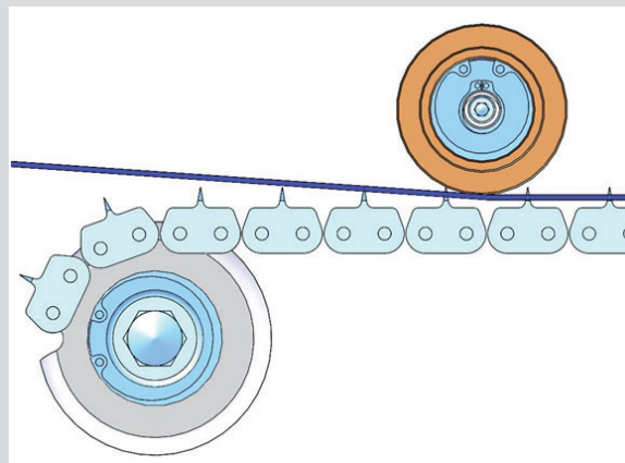
Neues Einstachel-Verfahren
