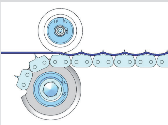
Altes Einstachel-Verfahren
